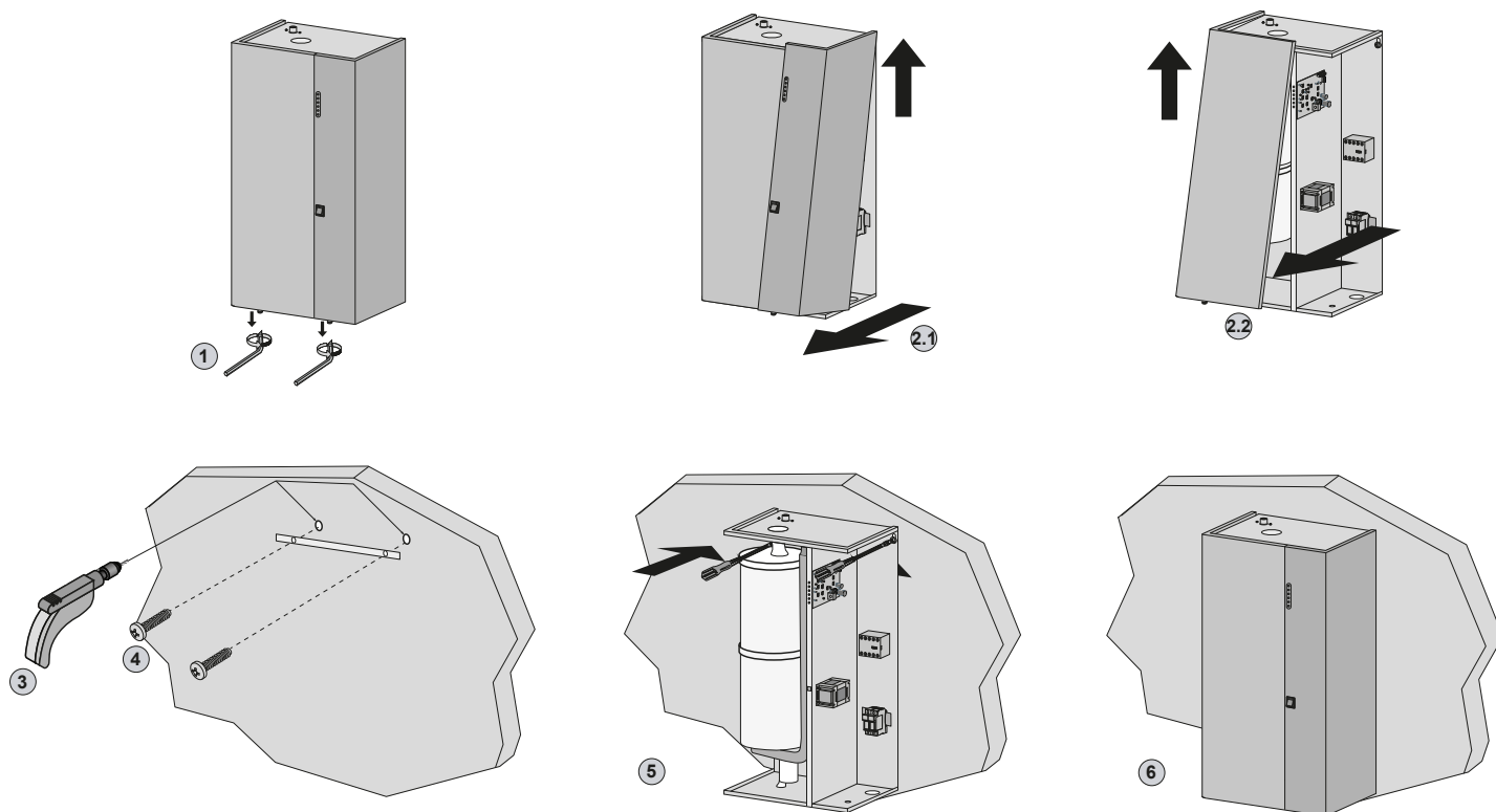
Fig. 3. Instructions de montage
