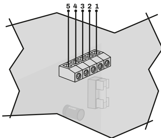
Fig. 19. Bornier auxiliaire M1
