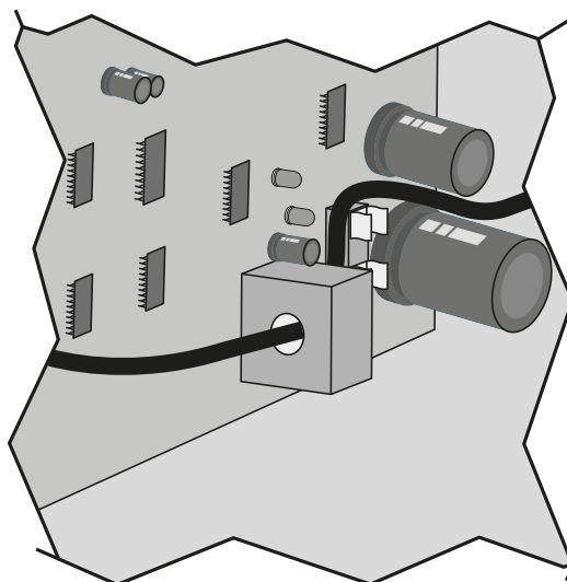
Fig. 26. Passage du câble à l'intérieur du TA
