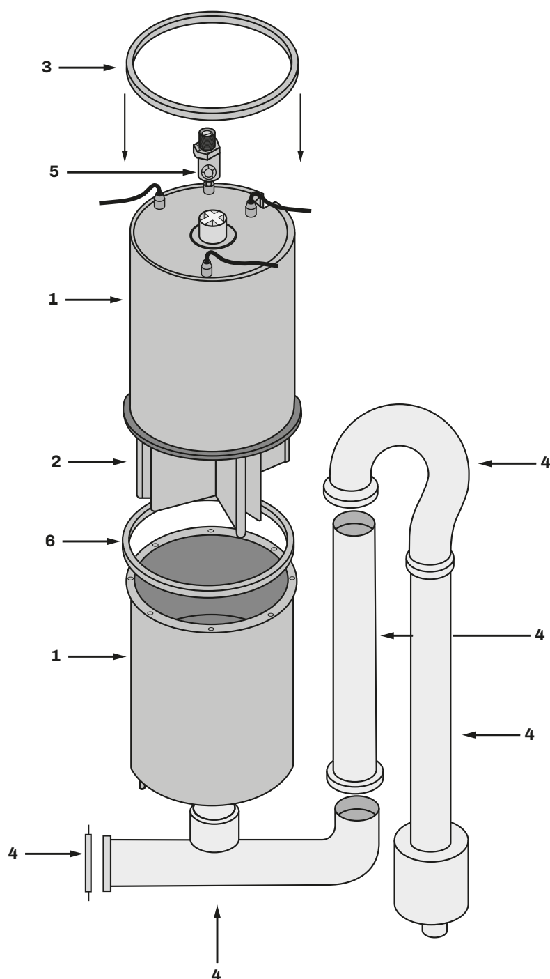
Fig. 27. Pièces de rechange Série KT - Partie hydraulique
