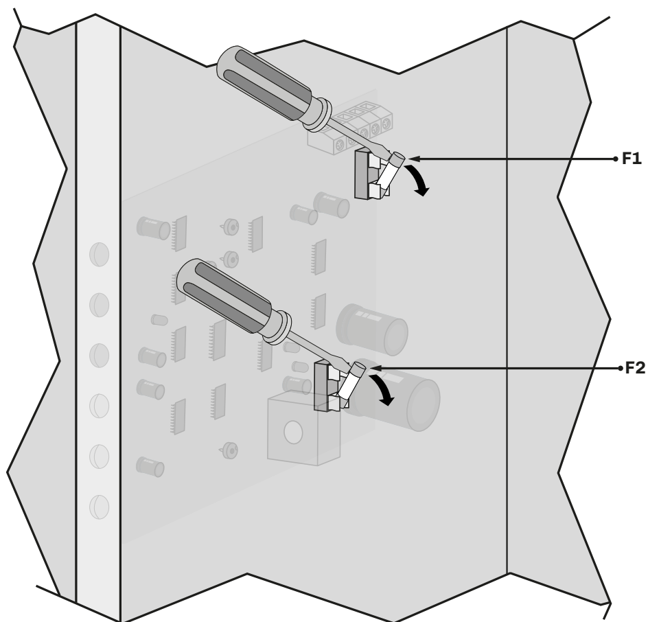
Fig. 18. Dispositifs de protection sur carte de contrôle
