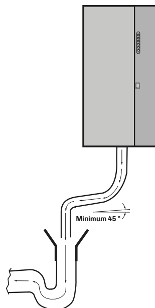
Fig. 4. Caractéristiques tuyau de vidange
