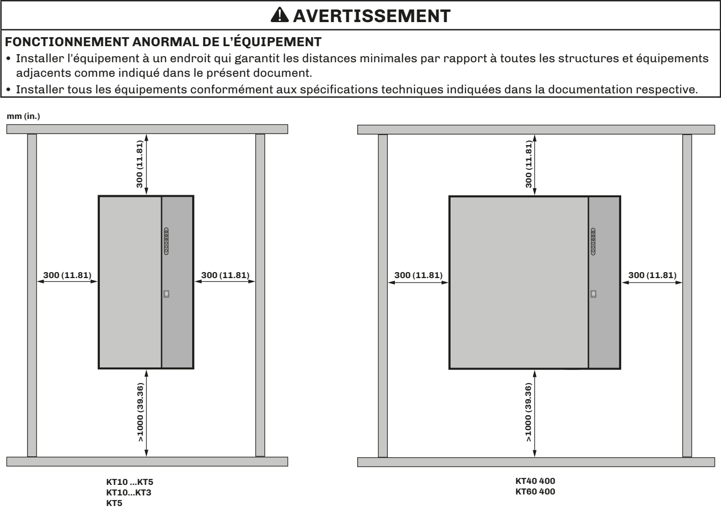
Fig. 2. Distances minimales de montage
