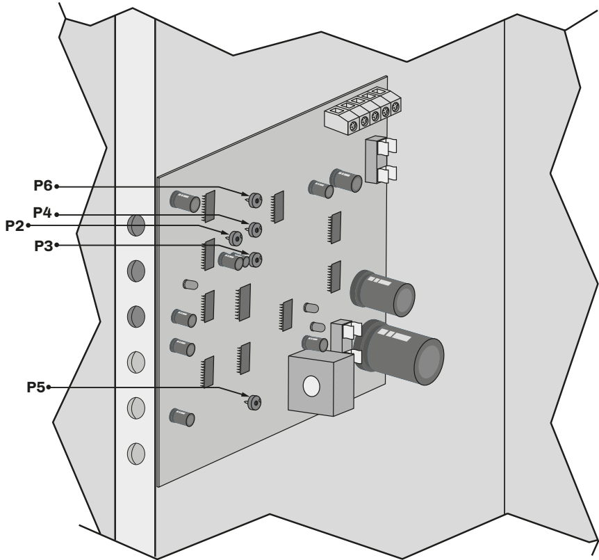
Fig. 25. Position potentiomètres
