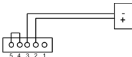
Fig. 21. Schéma de connexion avec hygromat avec sortie sous tension, ON/OFF et proportionnelle
