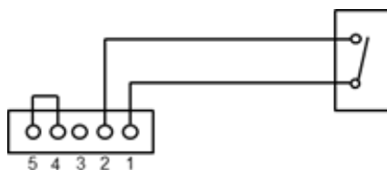
Fig. 20. Schéma de connexion avec hygromat ON/OFF
