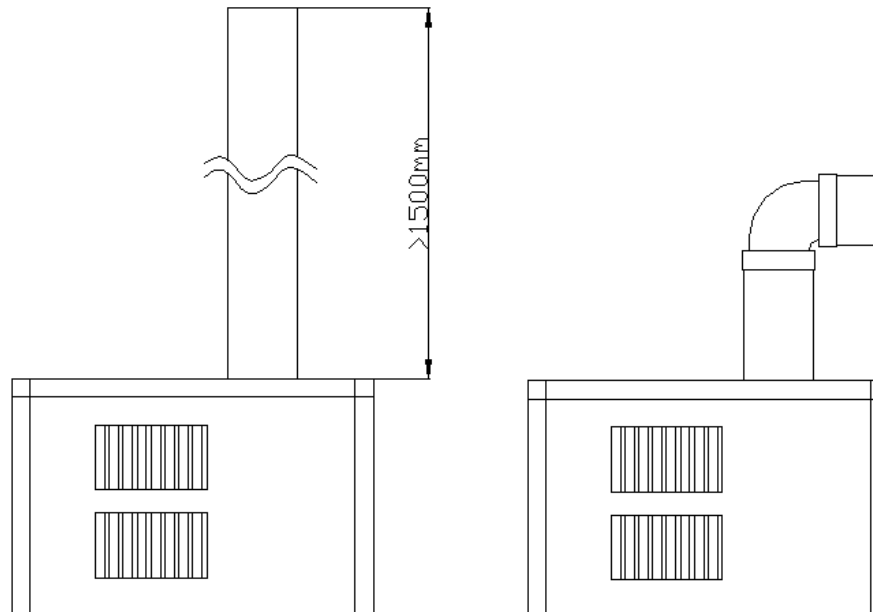
Figure 2 - Condotta uscita aria umida
