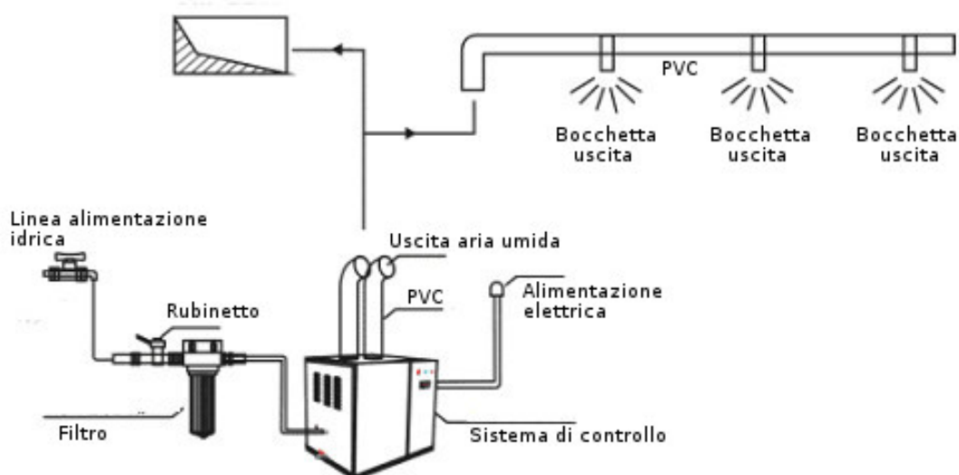
Figure 5 - Schema di istallazione
